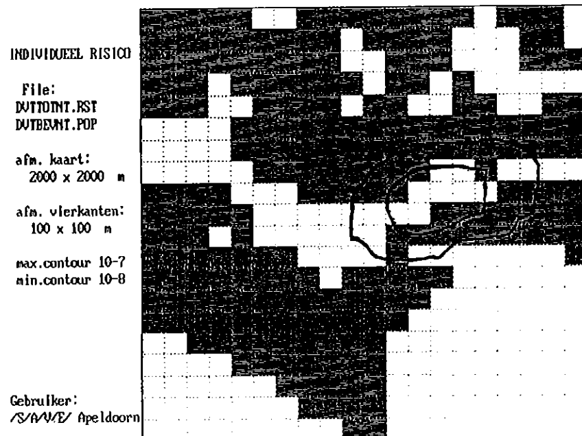
Figuur 7.2: Individueel risicocontouren (10 -7 -10 -8 ) ten gevolge van alle stoffen 1992
