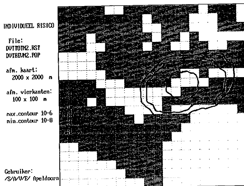
Figuur 7.6: Individueel risicocontouren ( 10^{-6} - 10^{-8} ) voor propaan 2010
