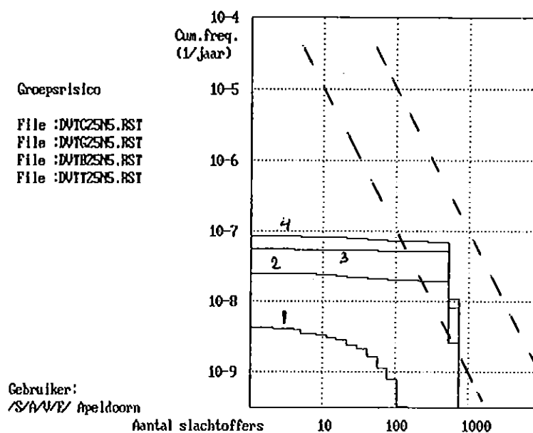
Figuur 9.1: Groepsrisico 1995, nachtsituatie (1 = chloor, 2 = propaan (gesloten), 3 = propaan (bont), 4 = totaal)
