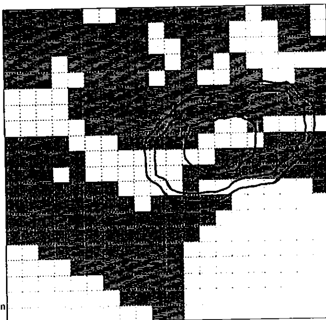
Figuur 7.7: Individueel risicocontouren ( 10^{-6} - 10^{-8} ) voor alle stoffen 2010
