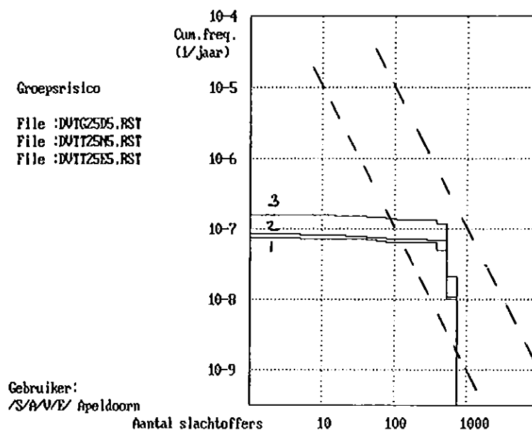
Figuur 9.2: Groepsrisico 1995 (1 = dag, 2 = nacht, 3 = etmaal)
