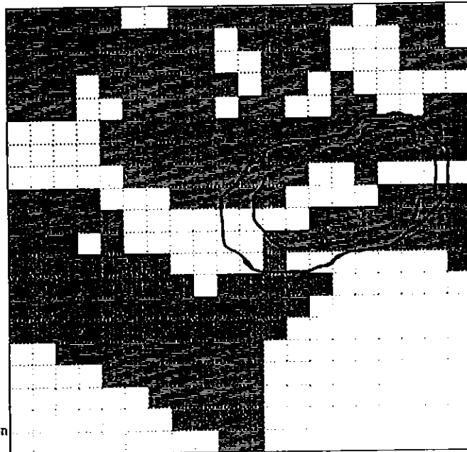
Figuur 7.3: Individueel risicocontouren (10 -7 -10 -8 ) voor propaan dagsituatie 2010
