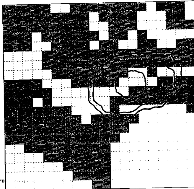
Figuur 7.4: Individueel risicocontouren (10 -6 -10 -8 ) voor propaan (bont vervoer) nachtsituatie 2010
