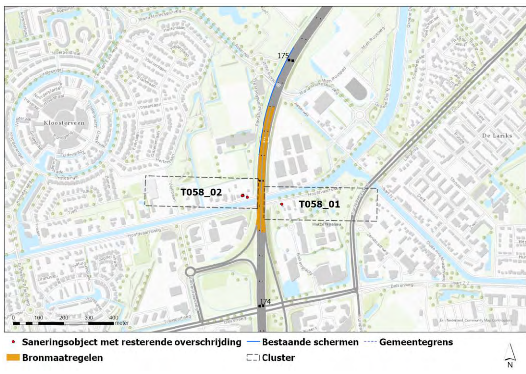
Figuur 20-1 Geluidbeperkende maatregelen gemeente Assen
