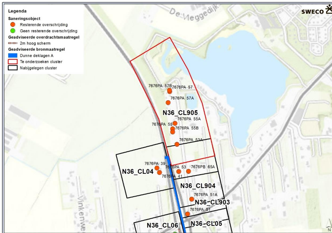
Figuur 171 Geadviseerde maatregelen (geen bron- en/of overdrachtsmaatregelen geadviseerd). De bronmaatregel aanwezig in de figuur hoort bij de nabijgelegen clusters N36_CL04t/m11+903+904.
