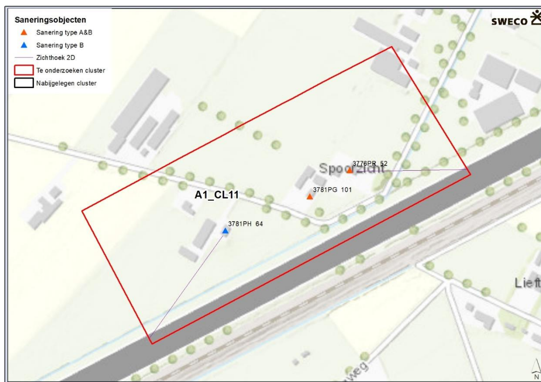
Figuur 3 Overzicht van cluster A1_CL11 (gemeente Barneveld)
