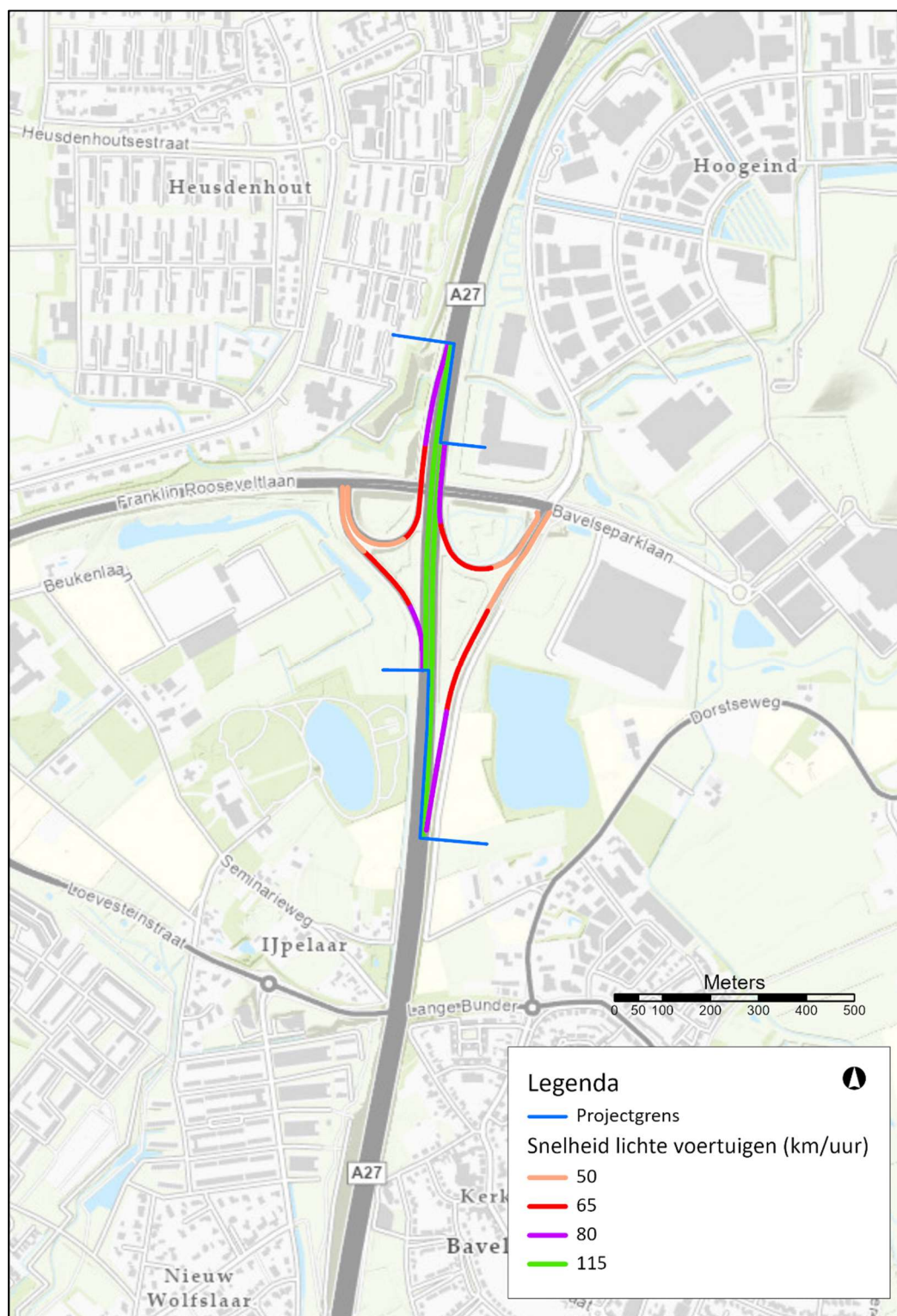
Figuur 7 Rijsnelheden per wegvak
