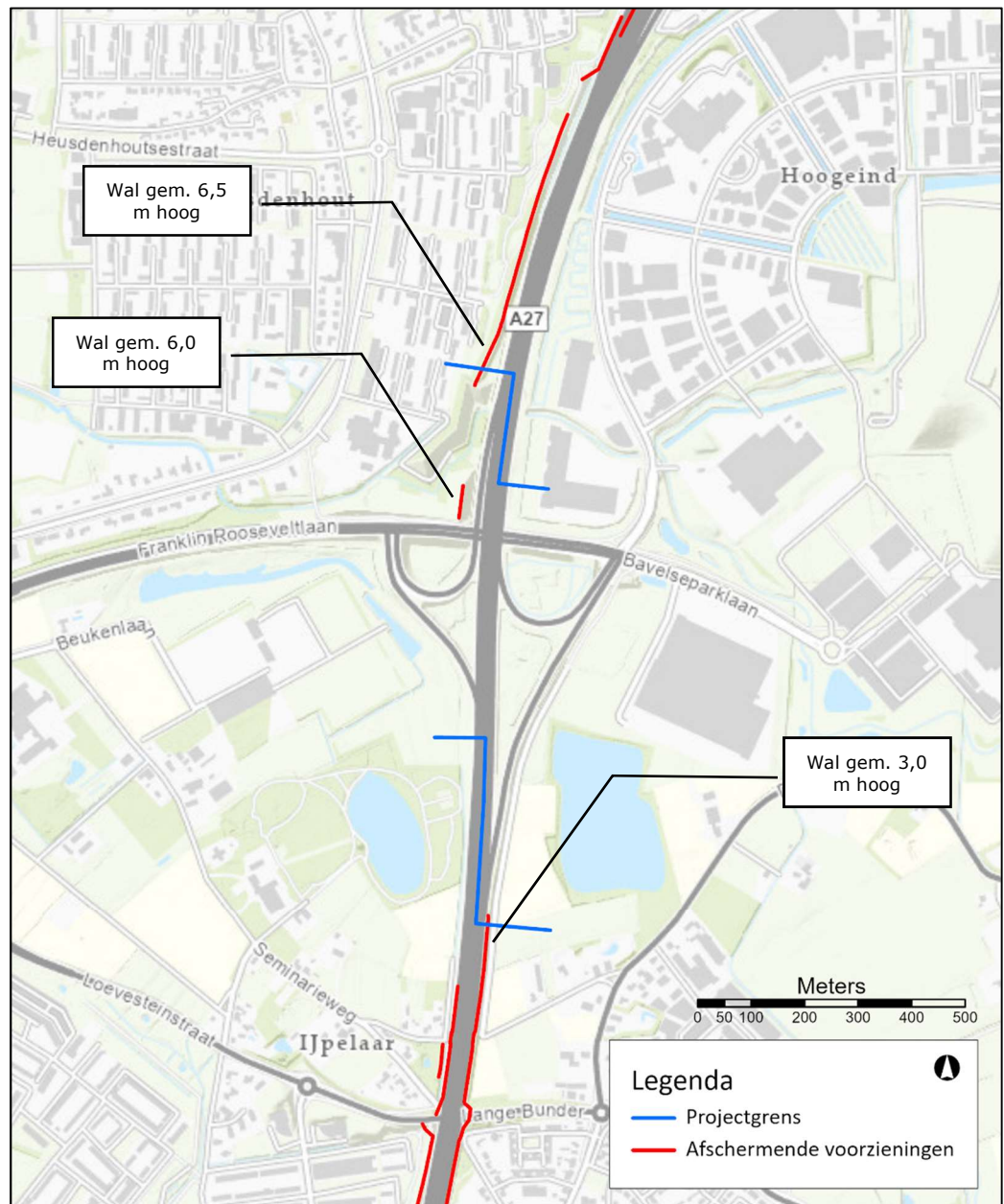
Figuur 10 Overzicht locatie geluidwallen Geluidregister
