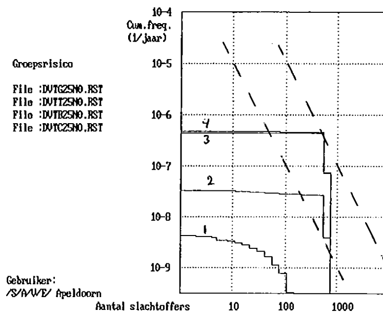
Figuur 9.3: Groepsrisico 2000, nachtsituatie
