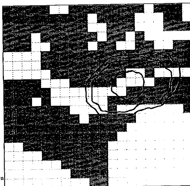
Figuur 7.6: Individueel risicocontouren ( 10^{-6} - 10^{-8} ) voor propaan 2010
