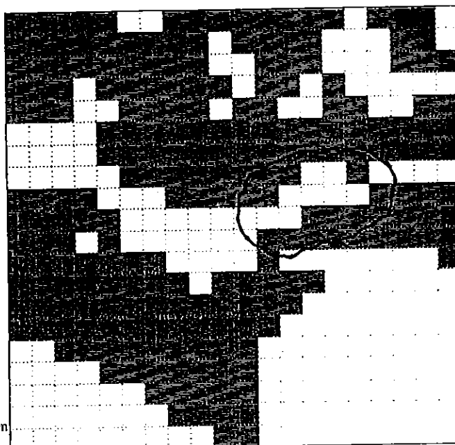
Figuur 7.5: Individueel risicocontour ( 10^{-8} ) voor propaan (gesloten vervoer) nachtsituatie 2010
