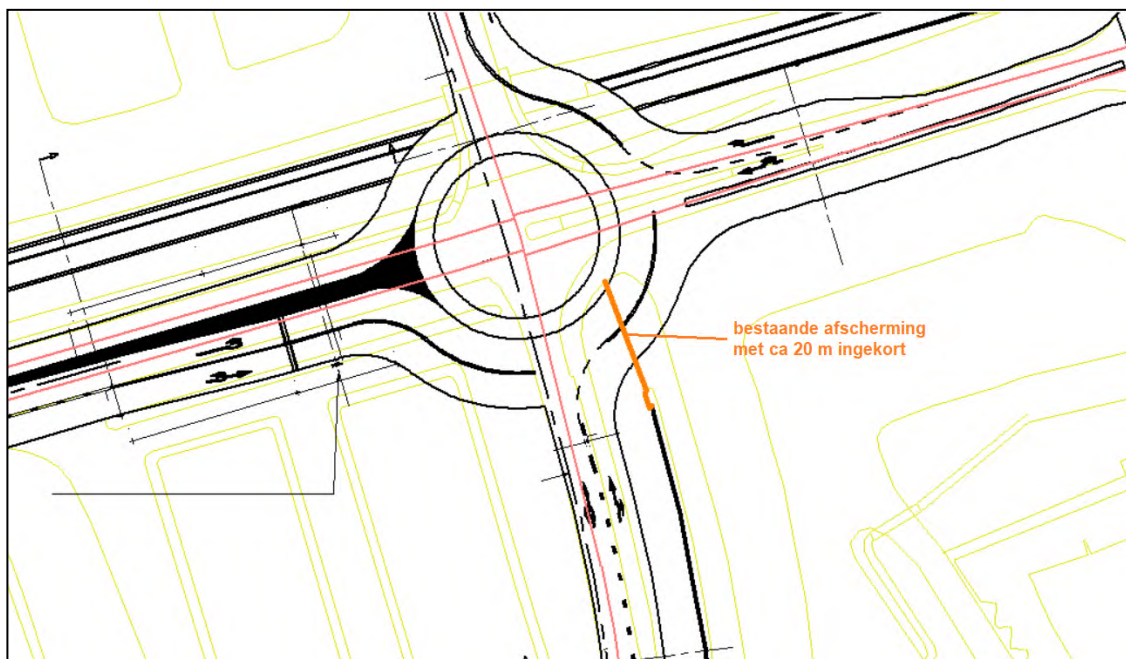
Figuur 6: Maatregelen oostelijke afrit
