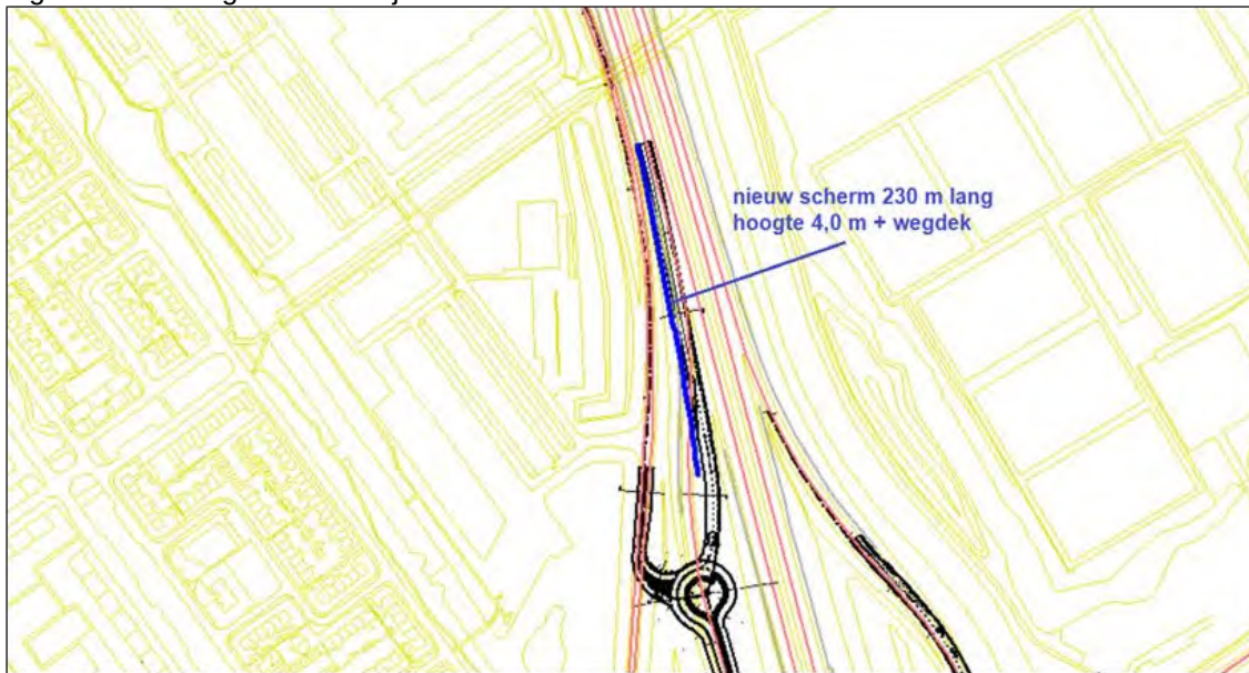
Figuur 5: Maatregelen westelijke afrit
