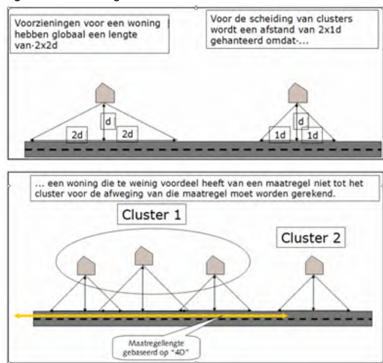
Figuur 6: Clustering
